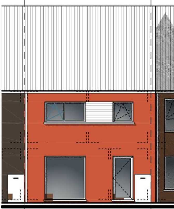
Façade Rue nord-est 1.100e
