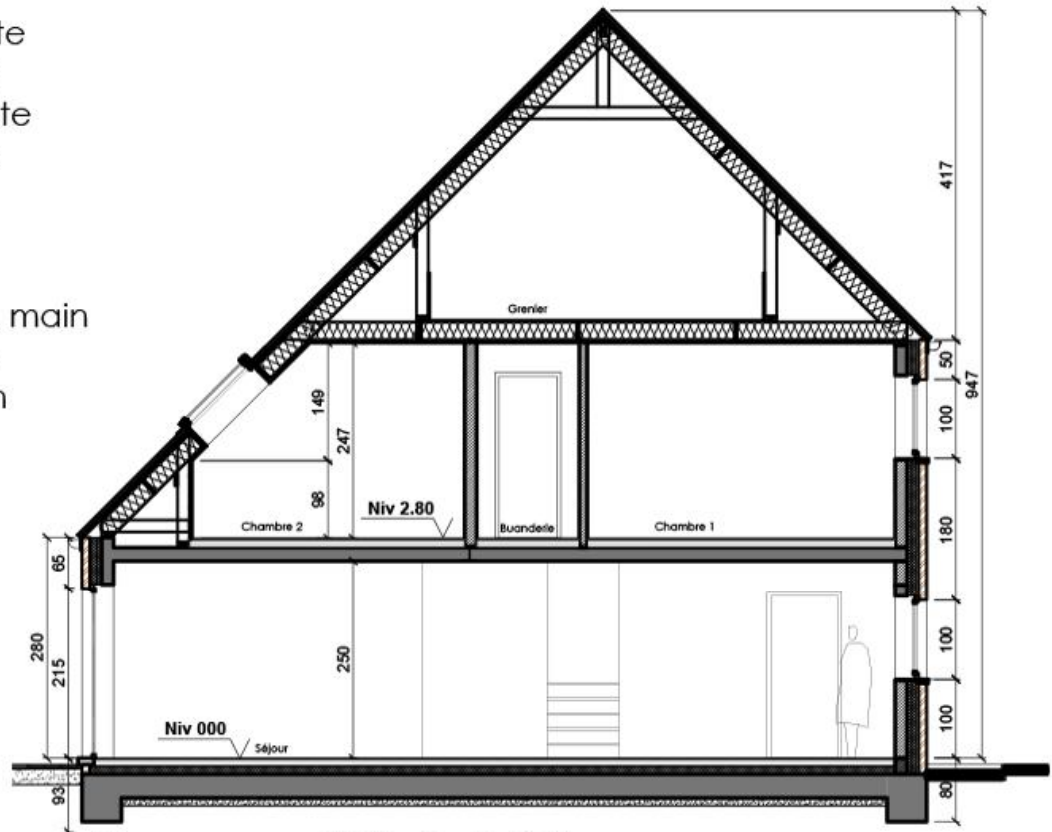
Coupe BB 1.100e
