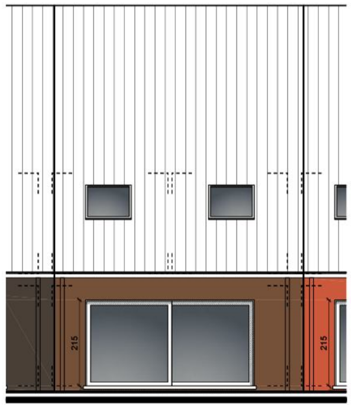
Façade Jardin sud-ouest 1.100e
