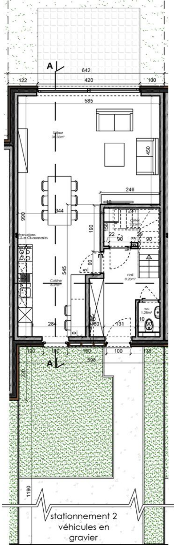
Plan RDC 1.100e
