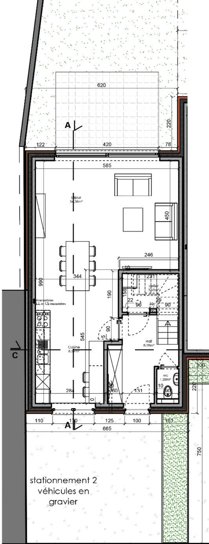
Plan RDC 1.100e
