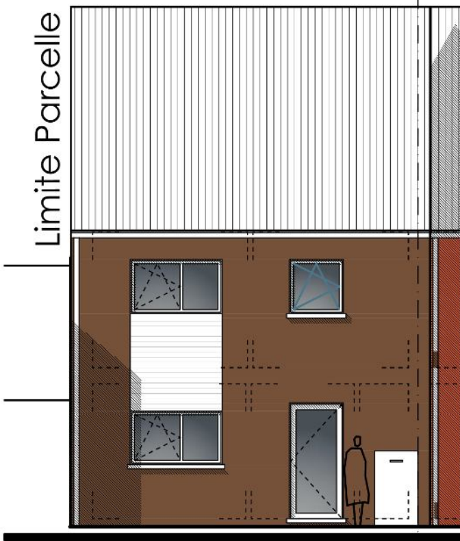
Façade Rue nord-est 1.100e
