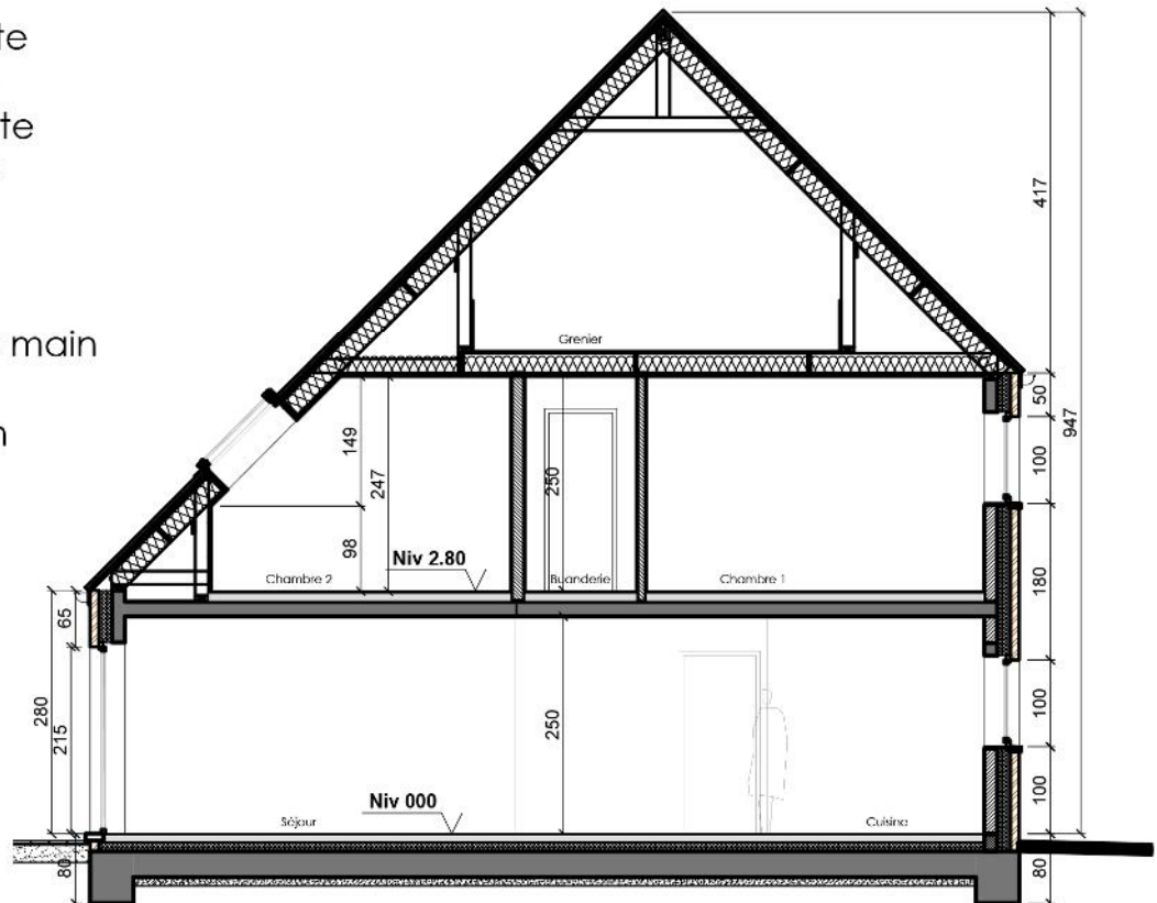
Coupe AA 1.100e
